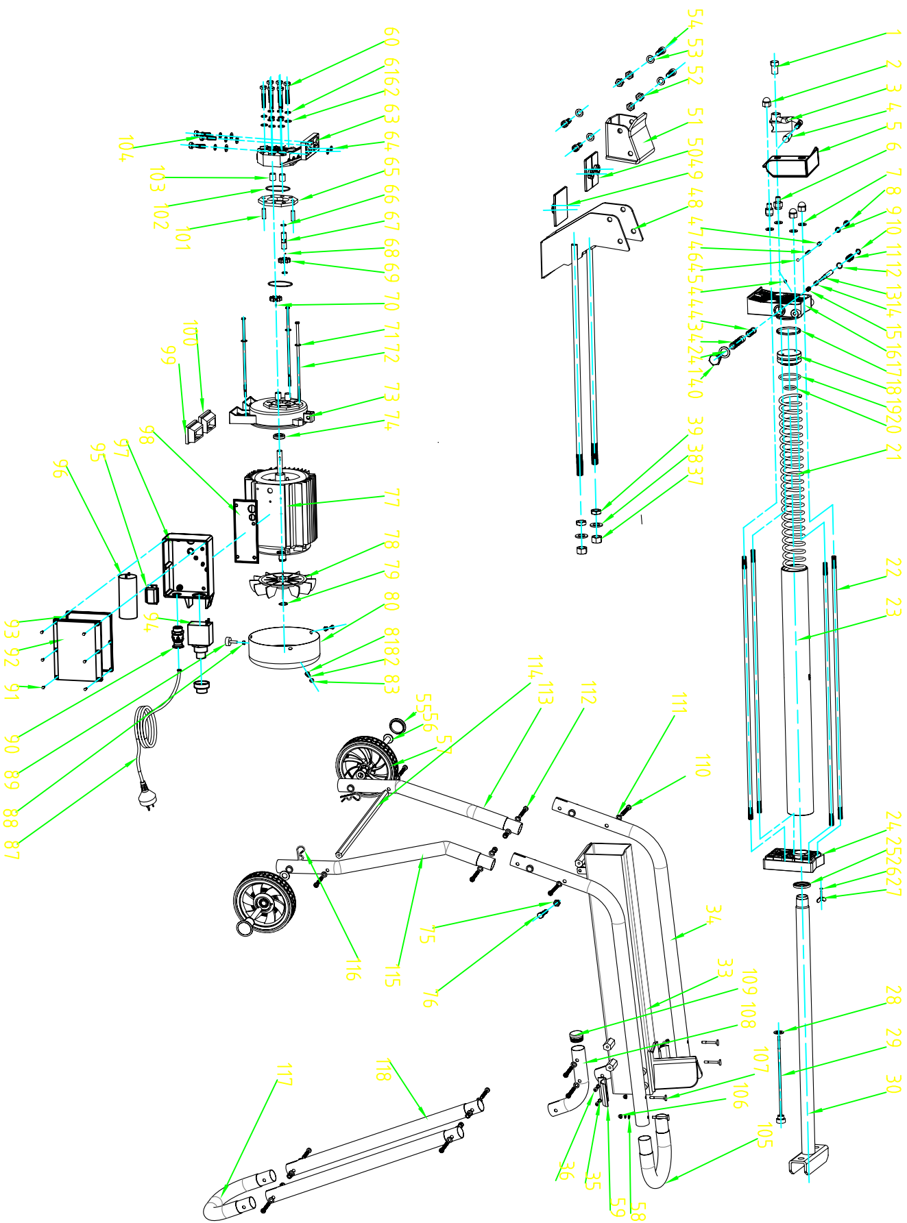
CBS8爆炸图
