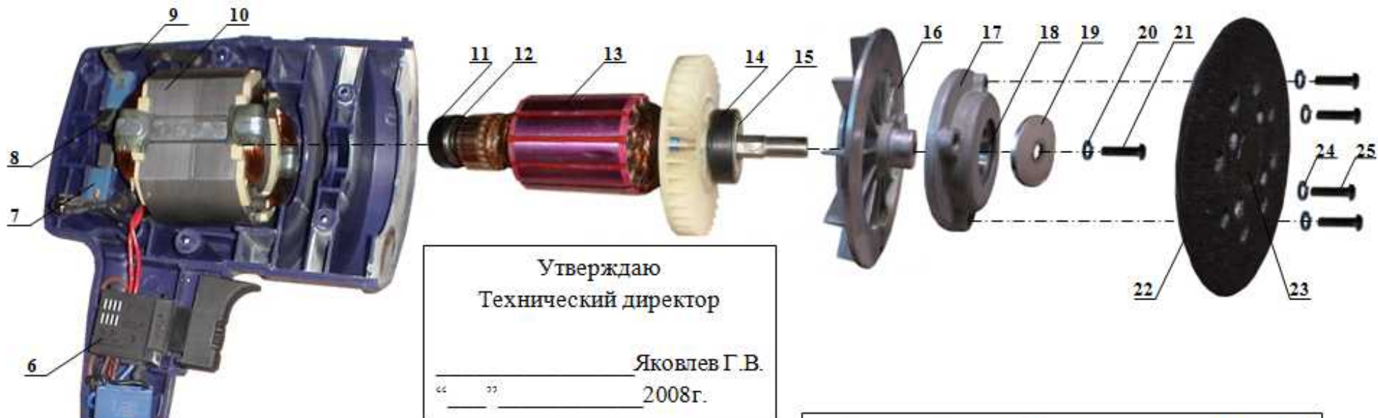
Машина полировальная электрическая МП-0,42
